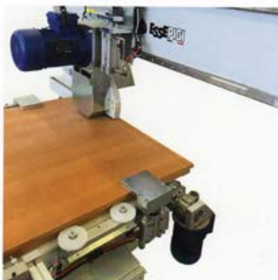
Taglio di pannello Panel cutting
